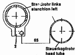
Ansicht B view B
